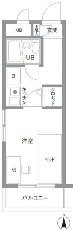
Aタイプ 18.72㎡ (5.66坪)
