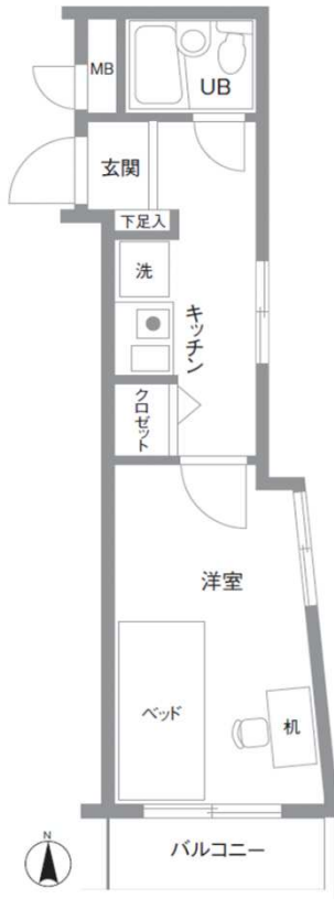
Dタイプ 20.55㎡ (6.22坪)
